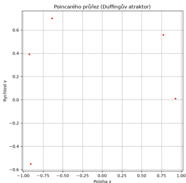
Obrázek 3: Poincarého průřez pro Duffingův oscilátor
